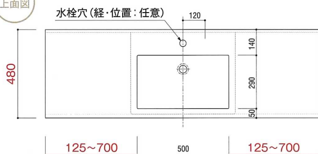
上面図
